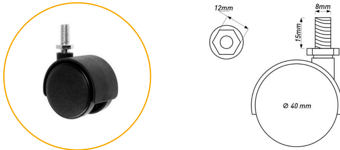
ОПОРА КОЛЁСНАЯ (НА РЕЗЬБЕ)
