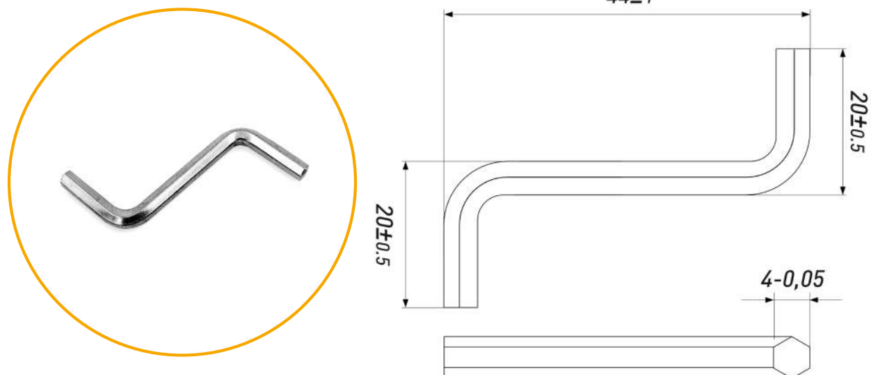
КЛЮЧ М4
