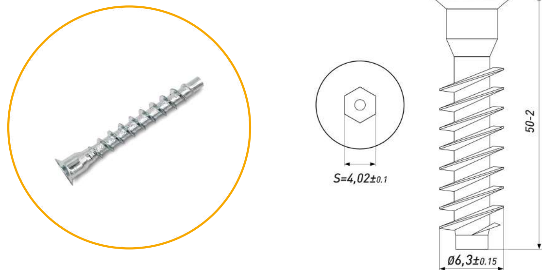
ЕВРОВИНТ 6,3*50
