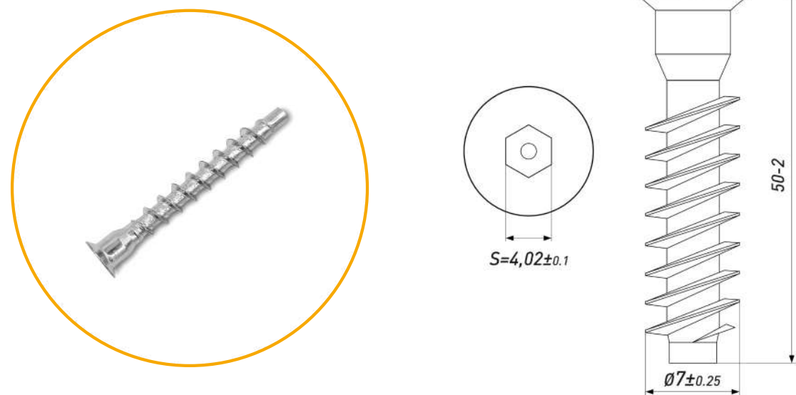
ЕВРОВИНТ 7*50
