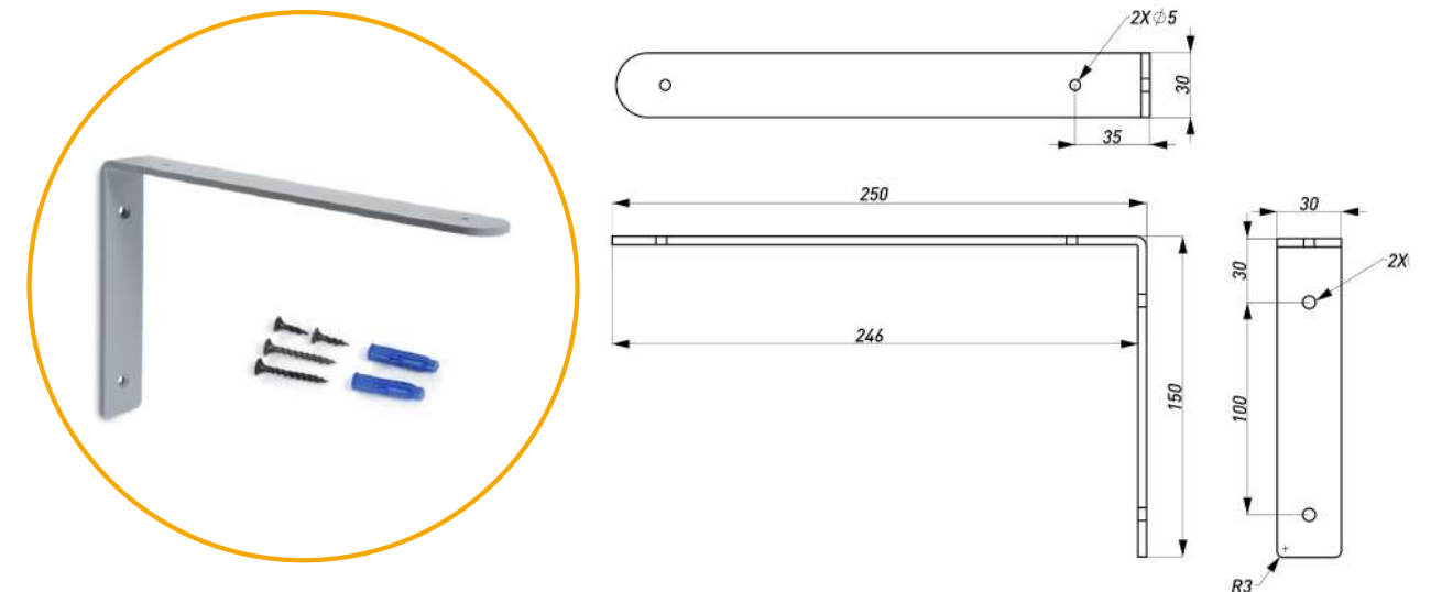
ПОЛКОДЕРЖАТЕЛЬ 1-01
