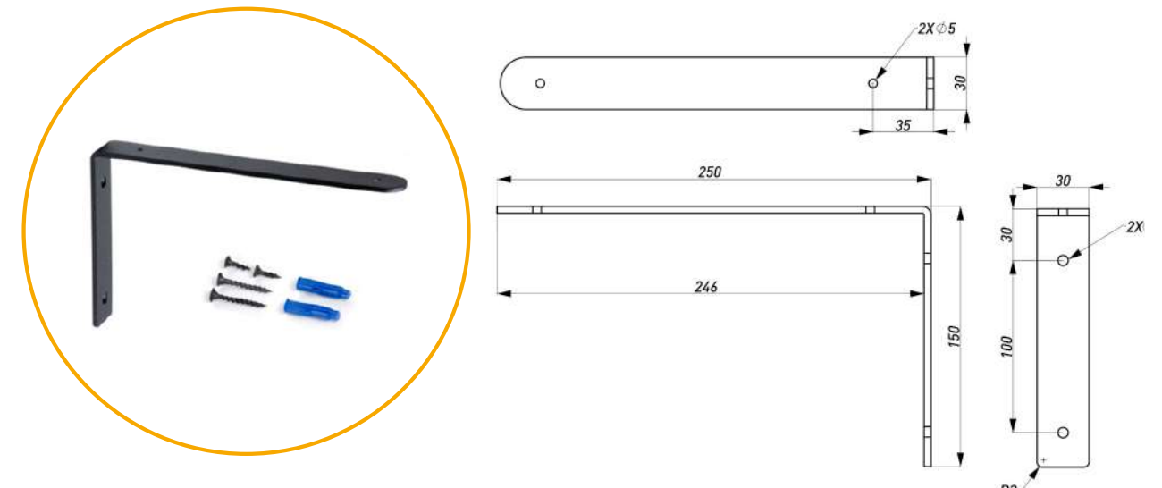
ПОЛКОДЕРЖАТЕЛЬ 1-01
