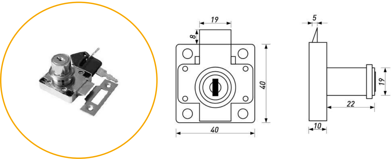
ЗАМОК МЕБЕЛЬНЫЙ № 338
