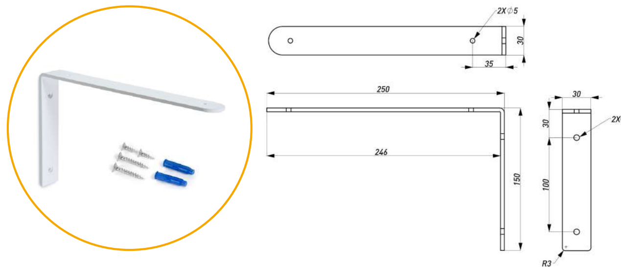
ПОЛКОДЕРЖАТЕЛЬ 1-01
