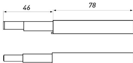
АМОРТИЗАТОР НАКЛАДНОЙ
